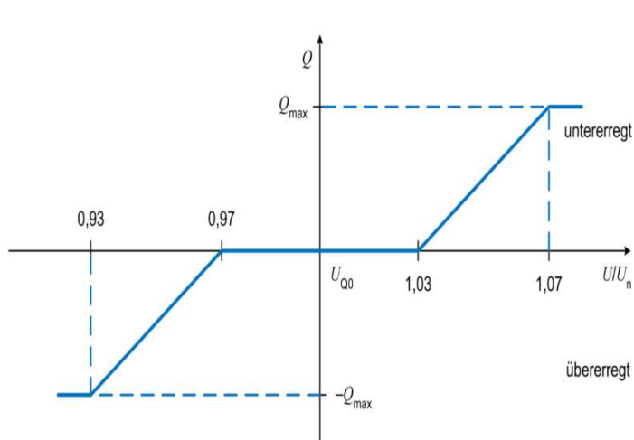
Bild 7 – Standard-Q(U)-Kennlinie
